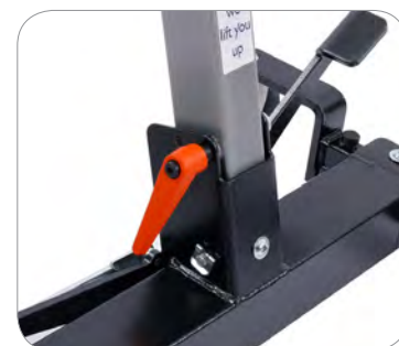
Schnellspannschraube zum werkzeuglosen Zerlegen des Lifters
